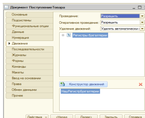
Рис.2 –Окно документа «Поступление Товара»
