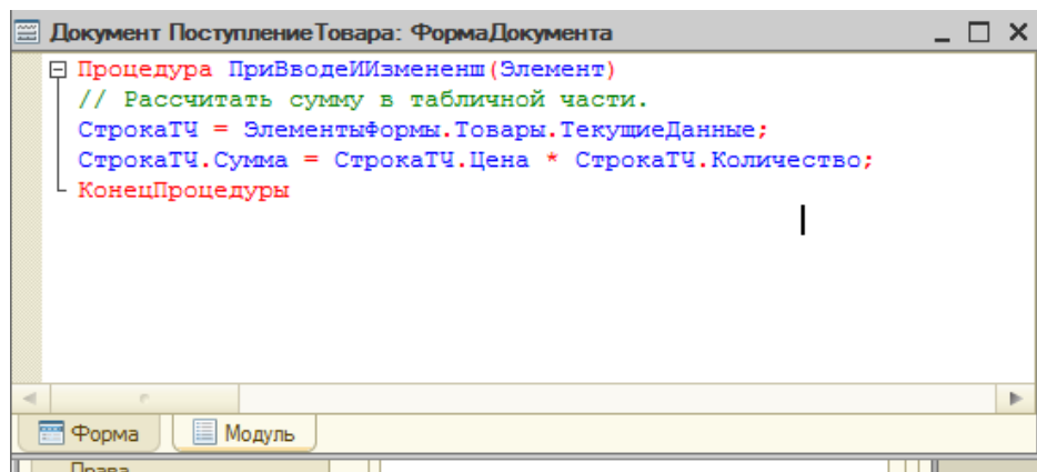
Рис.5 – Окно «Модуль» (Форма документа)
