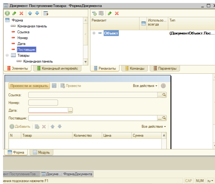
Рис.4 – Форма документа «ПоступлениеТовара»
